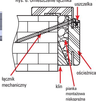
Rys. 6. Umieszczenie łącznika
