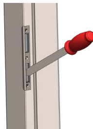
Rys. 7. regulacja zaczepu
