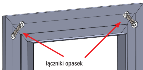
Rys. 9. Domykanie ościeżnicy bramką z kątowników
